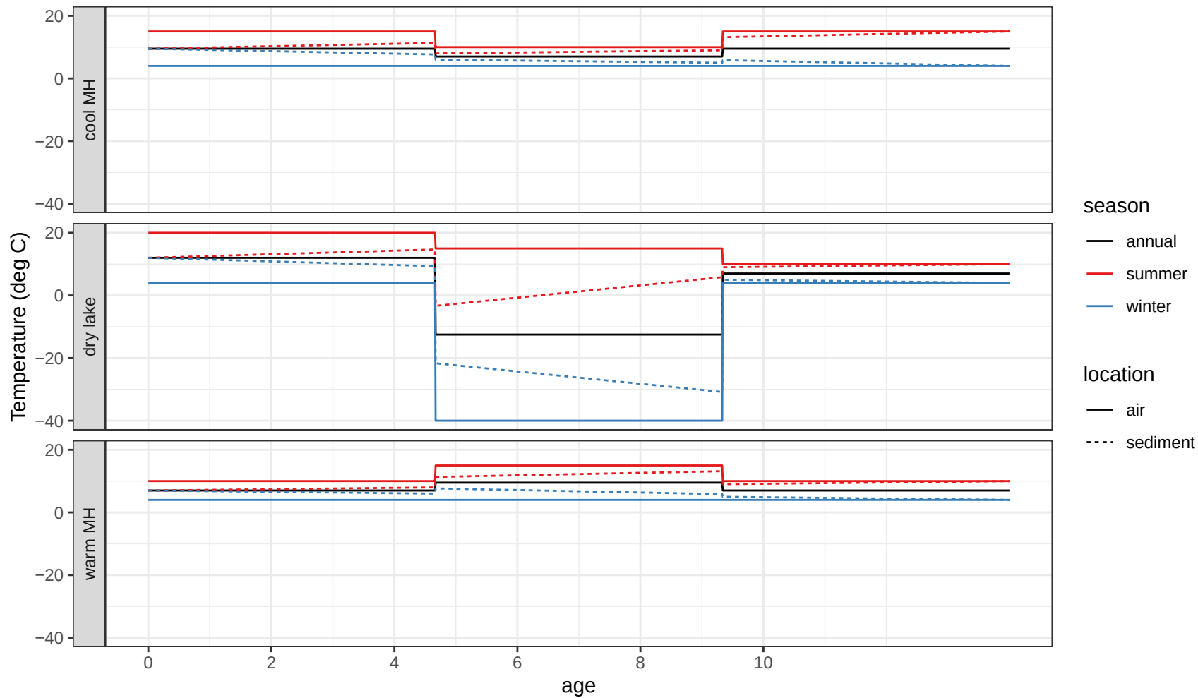
Simulated temperature trends. Holocene Mean air Temp = 2.16666666666653 deg C
